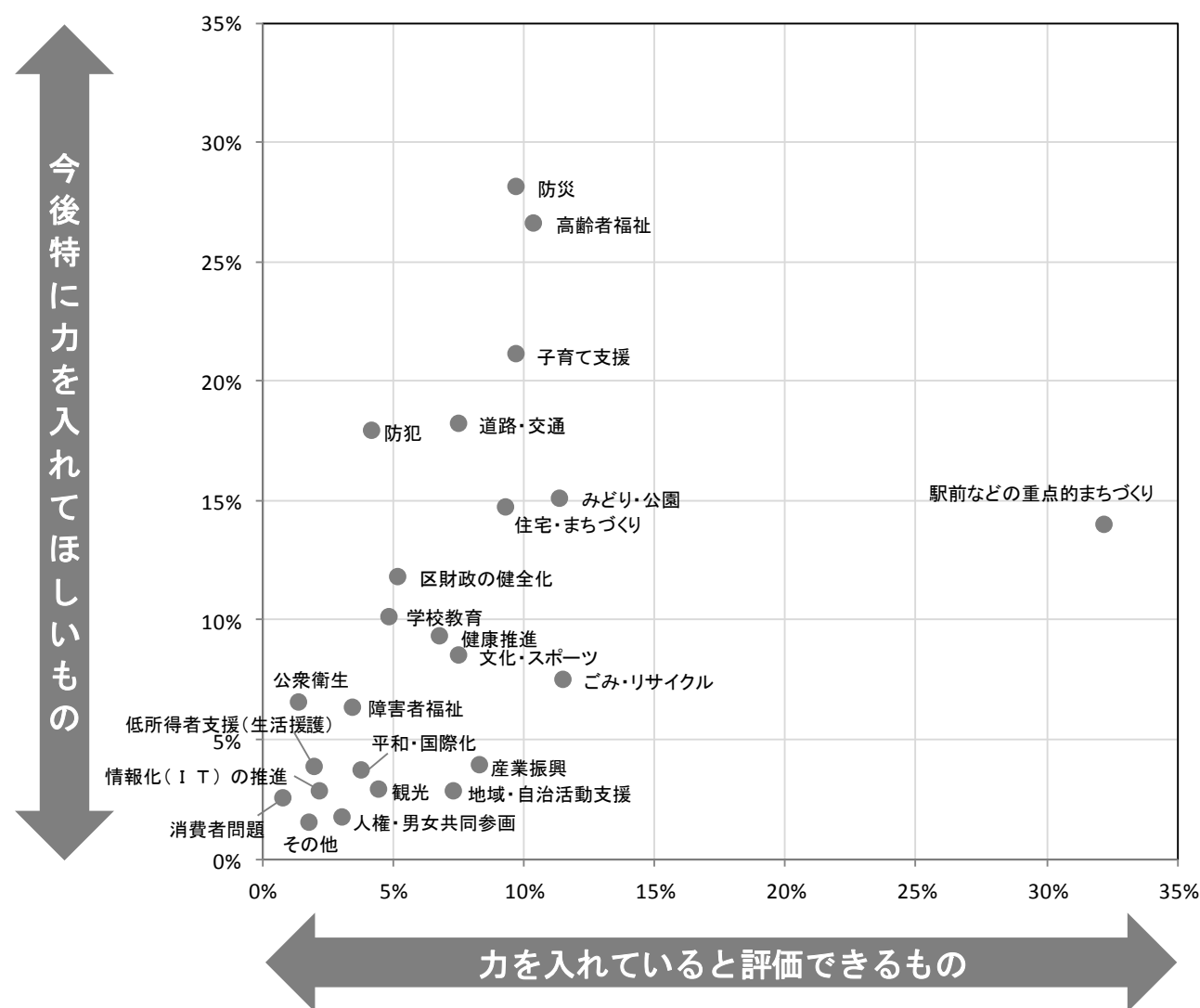
区の施策への評価と要望 散布図
